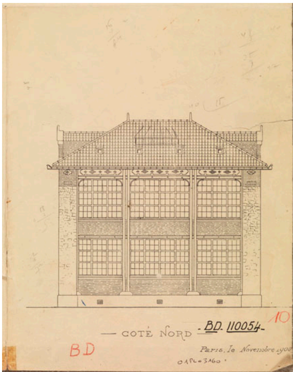
Elevation dressée par Paul Friesé le 1er novembre 1900. Bâtiment de l'administration, façade coté nord.
