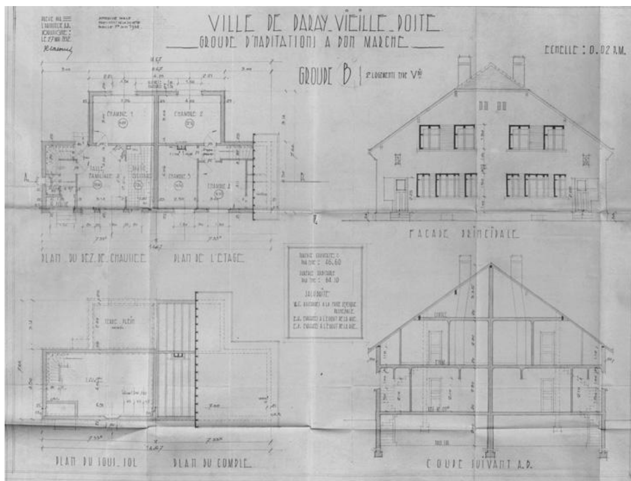
Pavillons du groupe B (2 logements du type Vbis : 64, 10 m2) : élévation principale, plans et coupe. 1er juin 1932.
