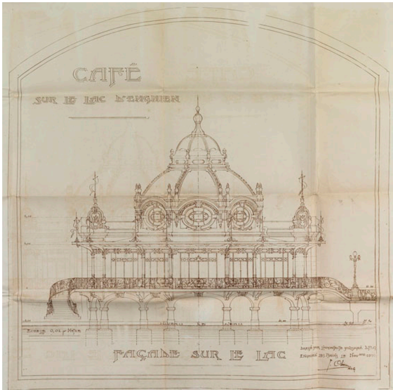
Élévation de la façade sur le lac, 1910. (AM Enghien-les-Bains, M1)
