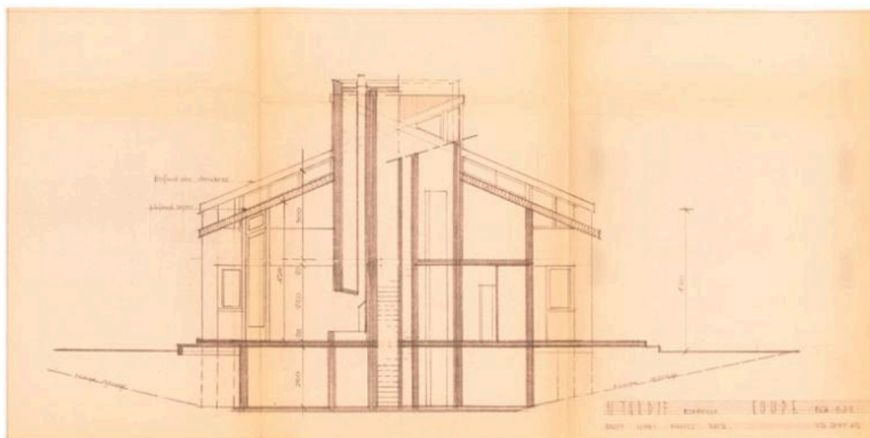
Coupe (extrait du permis de construire).
