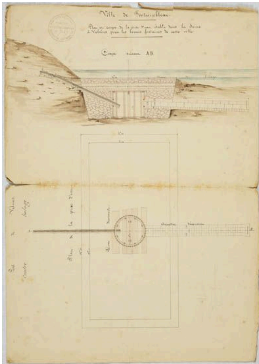
Plan et coupe de la prise d'eau établie à Valvins, en 1855, pour l'alimentation des bornes fontaines de Fontainebleau. (AD Seine-et-Marne, 3353W1169 )
