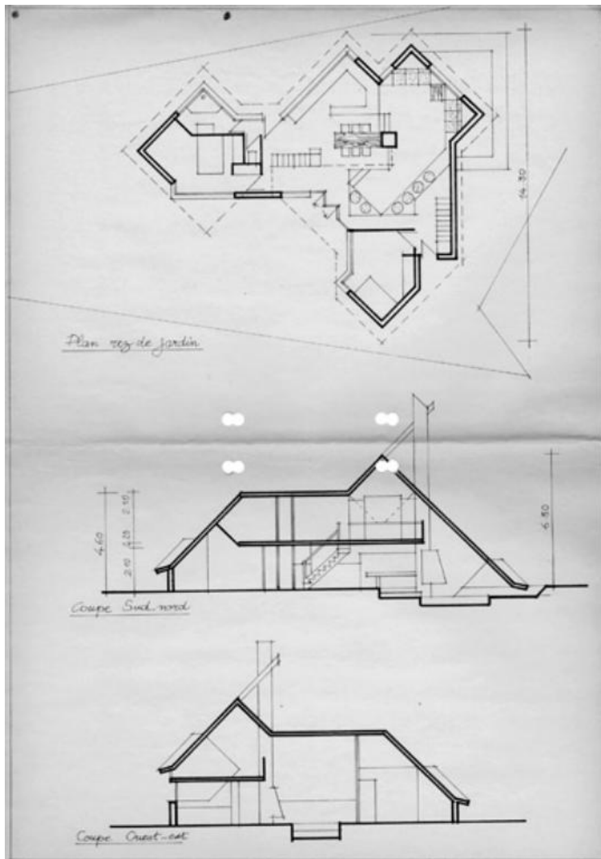
Plan et coupes, extrait du permis de construire.
