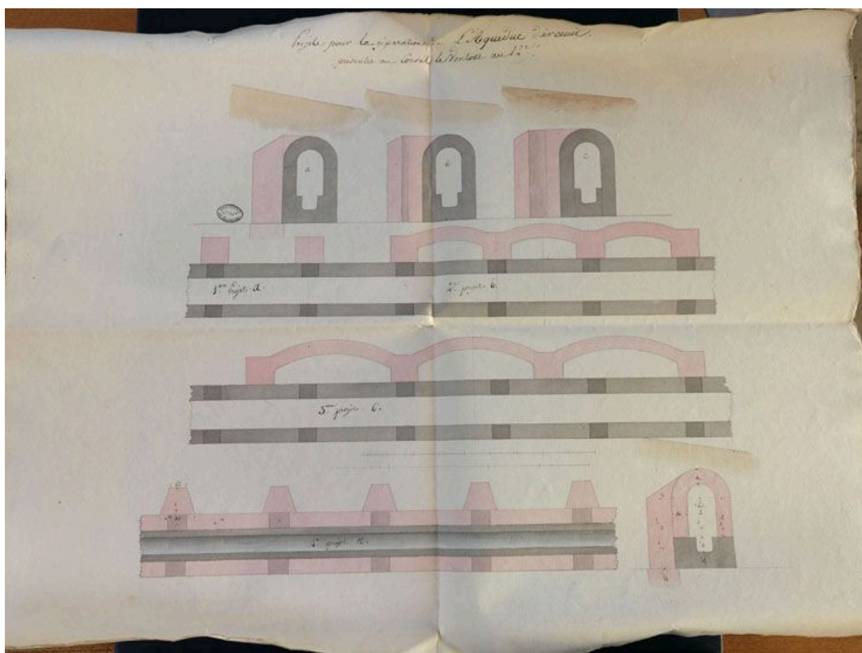
Arcueil. Coupe de la galerie pour réparation fin XVIIIe siècle début XIXe siècle. (AN, F/13/1004)
