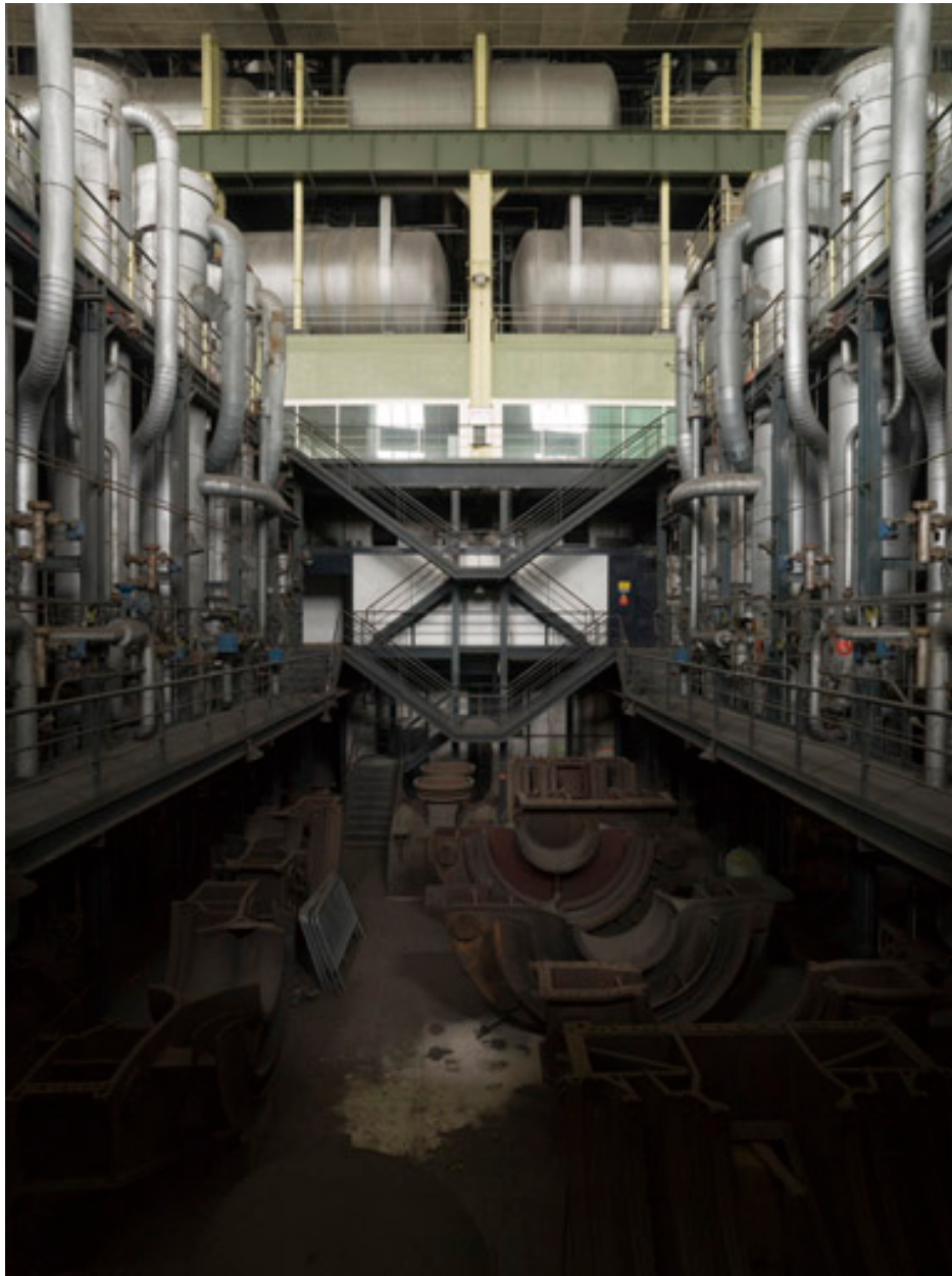
Poste d'eau tranche 125 MW. Turbines
