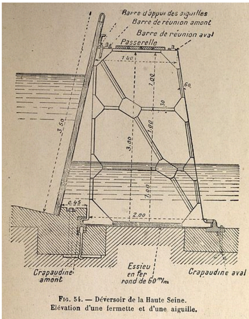
Déversoir de la Haute Seine. Elévation d'une fermette et d'une aiguille. Tiré de : Notions de navigation intérieure / M. Fourrey. Paris : Ecole spéciale des travaux publics, 1929.
