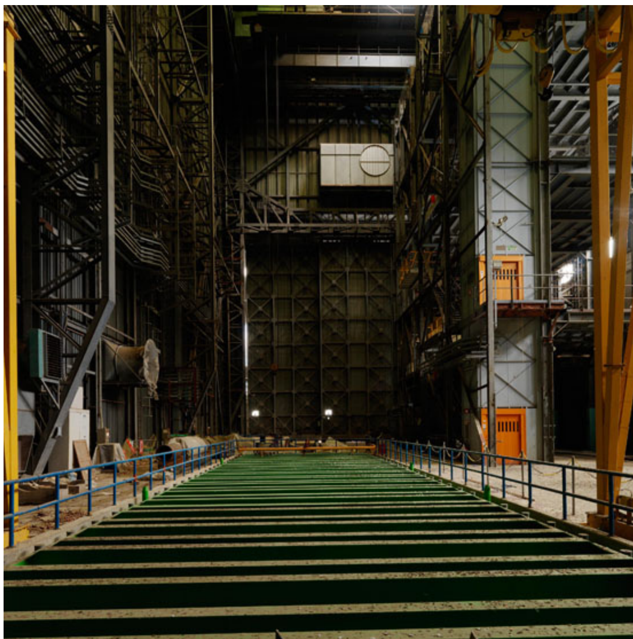
Intérieur du Hall CGVS (Circuit d'essais de Générateurs de Vapeur chauffés au Sodium).
