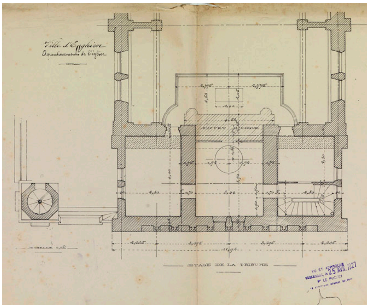
Agrandissement par la façade : plan de l'étage au niveau de la tribune, 1927. (AM Enghien-les-Bains, M48)
