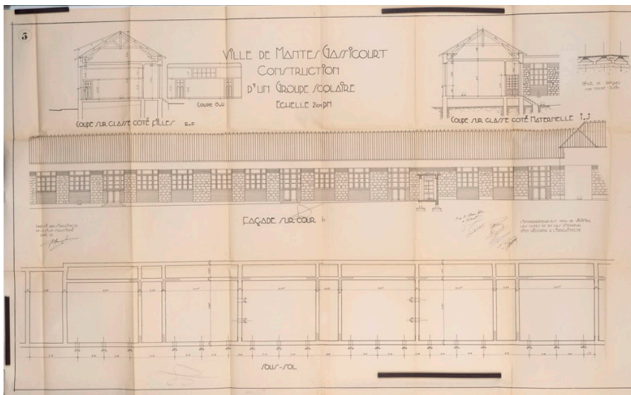
Façade sur cour et coupes. Marabout. 1932 (AM Mantes-la-Jolie 5 M 15 (2))
