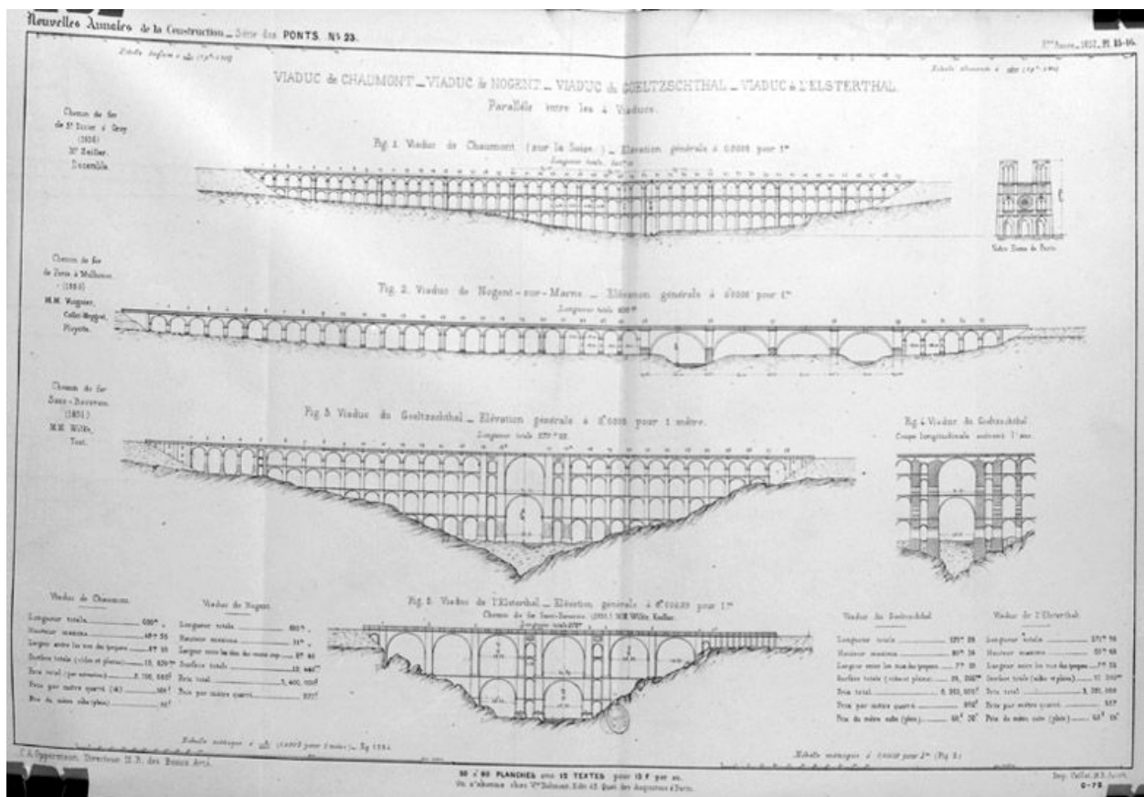
Elévation générale. Tiré de : Nouvelles annales de la construction, 1857. (
