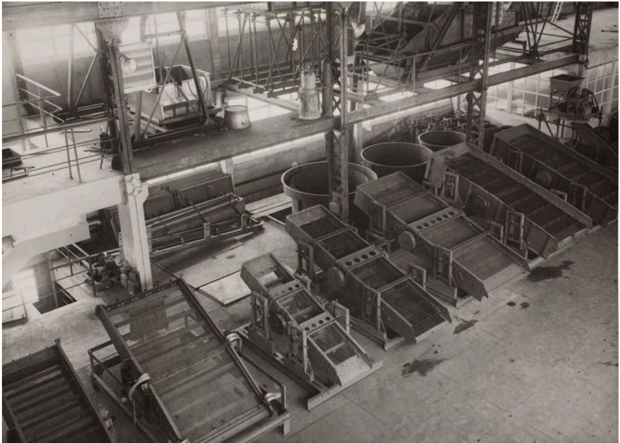
Vue intérieure de la station d'essai des bureaux d'études PIC à Fontainebleau. Photographie. (AD Seine-et-Marne, 256J3)
