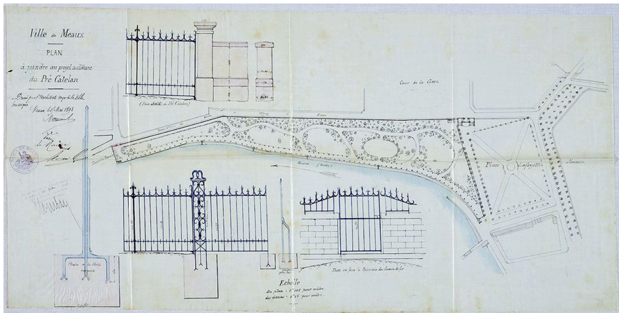
Plan pour projet de clôture du Pré Catelan (Jardin des Trinitaires), 1893. Calque. (AD Seine-et-Marne. 4 Op 284/16)
