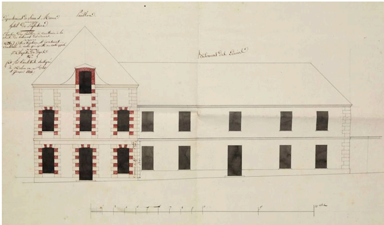
Élévation d'un pavillon à construire à la suite du bâtiment des écuries. Décembre 1820- janvier 1821. (AD Seine-et-Marne. 4 N 18-5)
