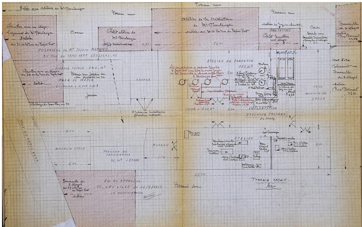
Plan du rez-de-chaussée, indiquant la fonction des ateliers et l'emplacement des équipements, 1968 (AD93 SC 7852).
