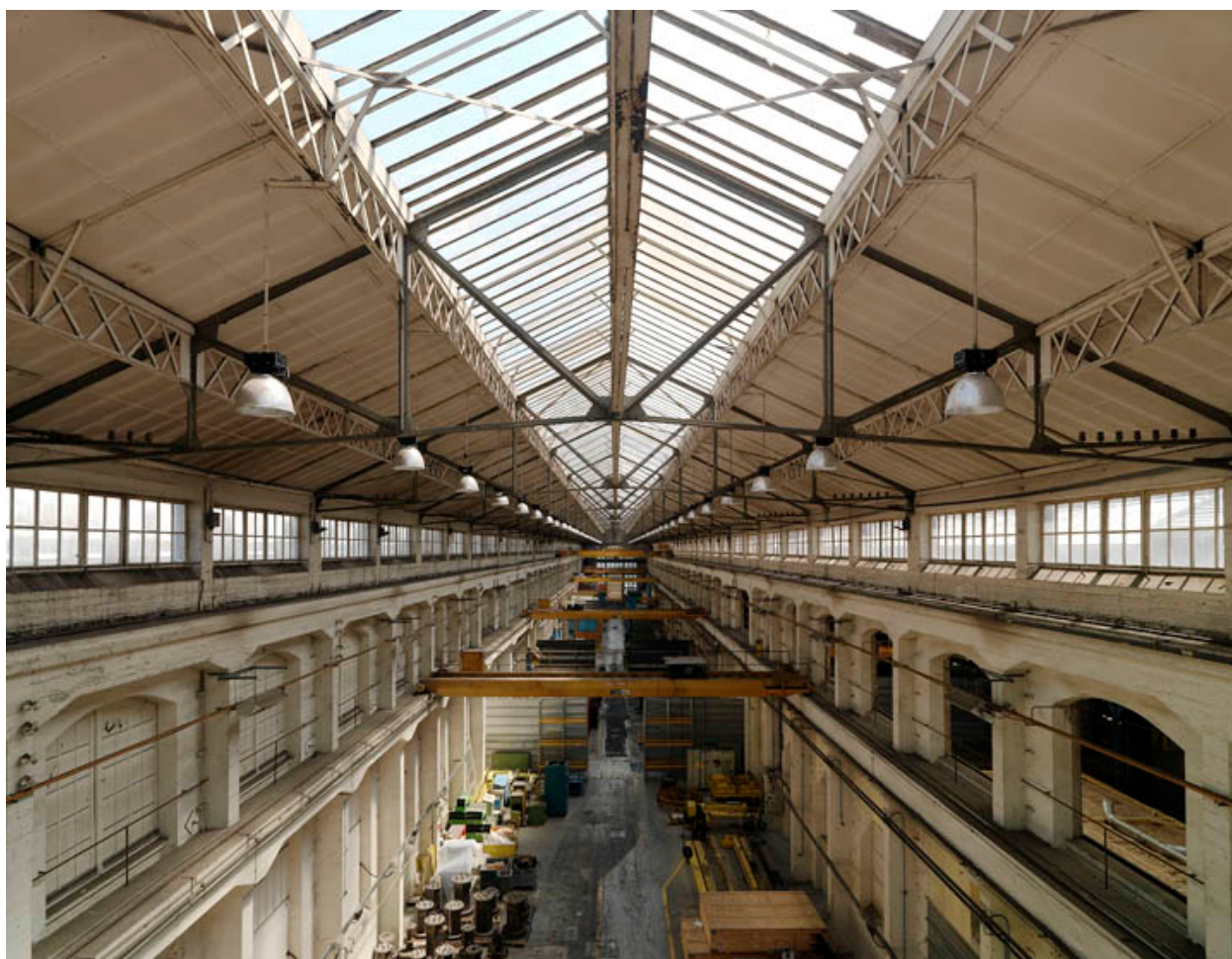
Vue intérieure. Liaison longitudinale nord. Ateliers d'armement puis de mécanique (1918). Actuellement entreprise Jeumont Electric. La verrière et la charpente métallique.
