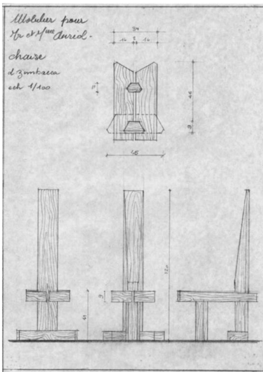
Dessin préparatoire pour la chaise "Joker".
