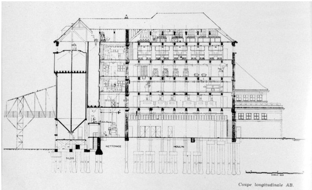
Coupe longitudinale AB. Photogravure, 1949. Tiré de : L'Architecture française, constructions industrielles (II), n° 85-86, 1949. (AM Melun. 578 W 3)
