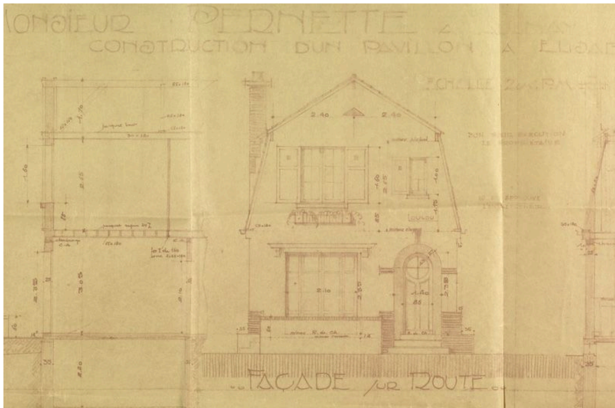
Elévation de la maison de Monsieur Pernette. Architecte : A. Schiketans, 1934 (AM Aubergenville).
