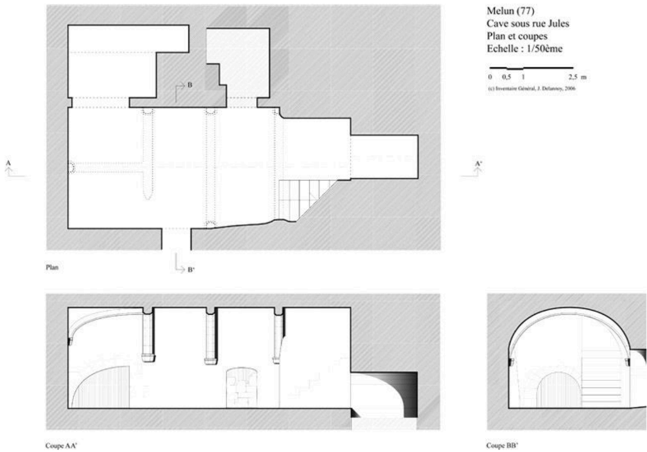
Plan et coupes de la cave.
