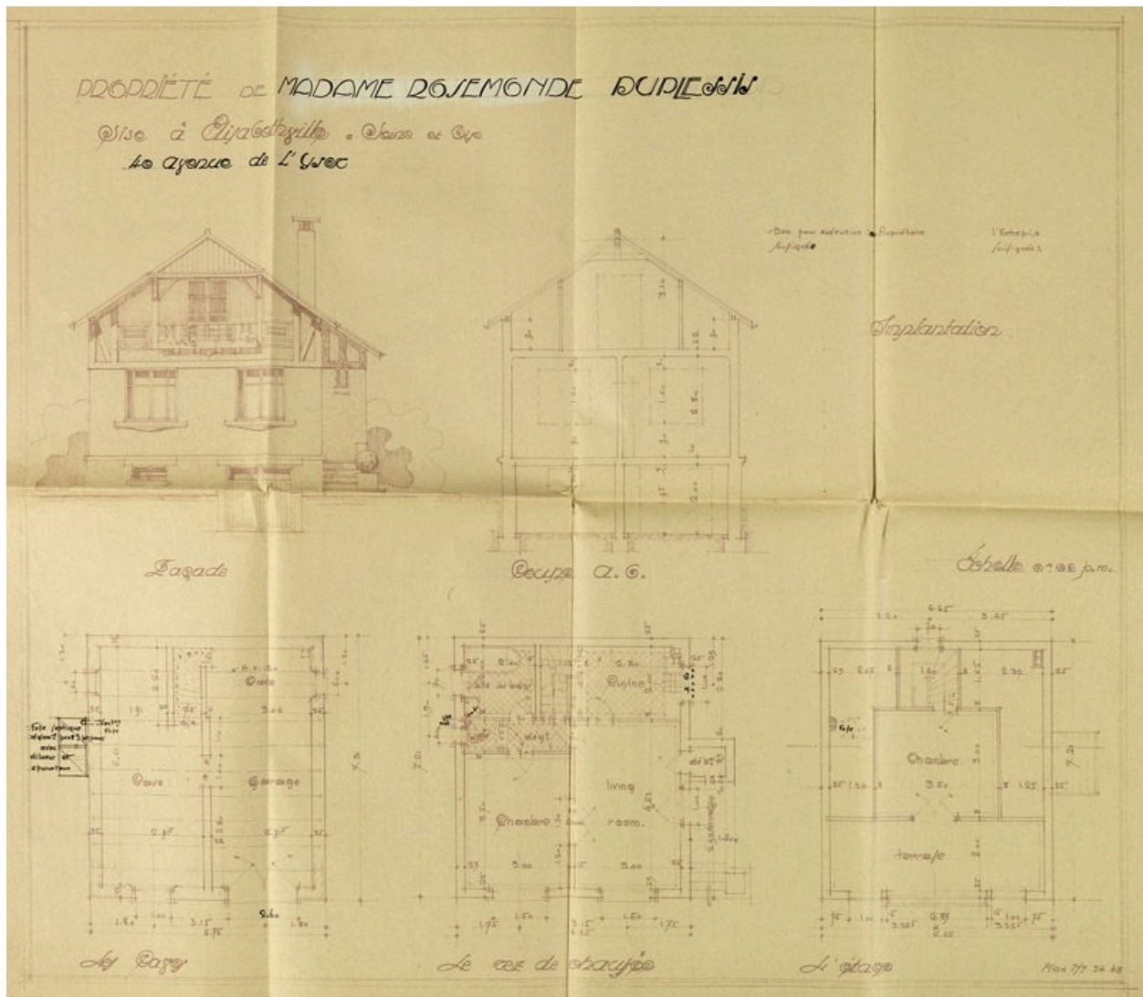
Plans de la maison de Mme Duplessis, 40 avenue de l'Yser. (AM Aubergenville).
