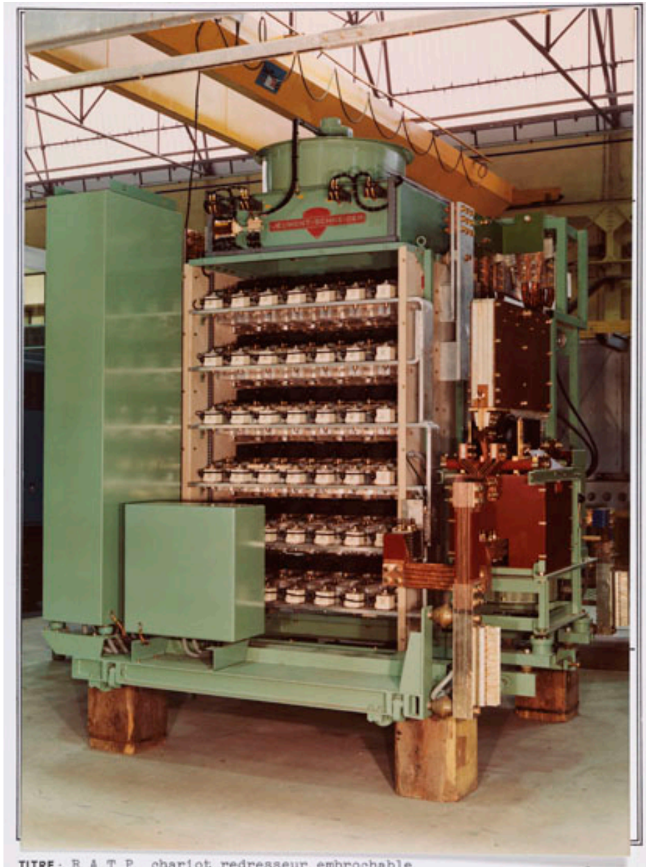
TITRE : R A T P - chariot redresseur embrochable
