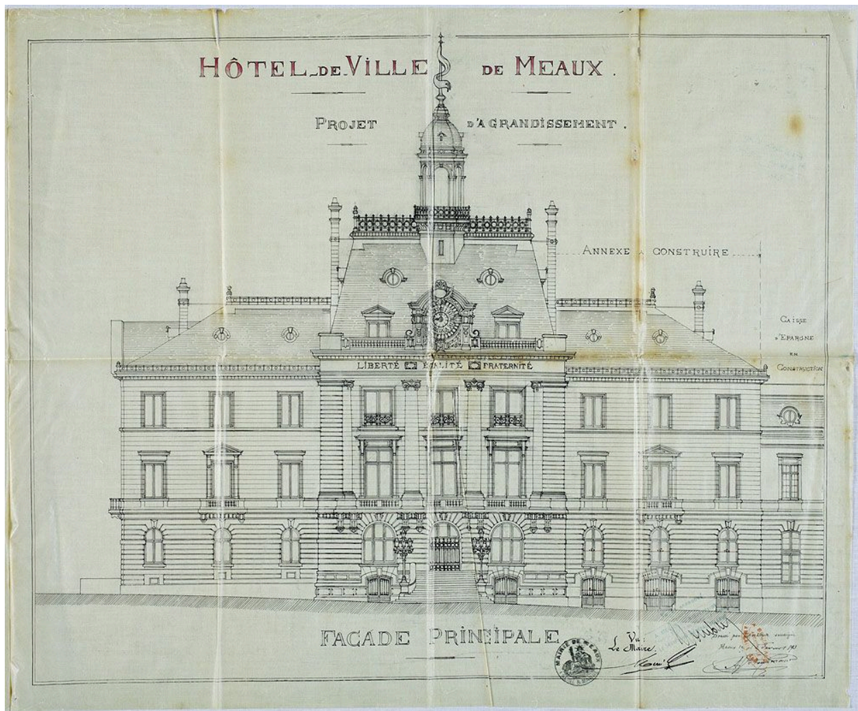
Projet d'agrandissement, 1893 : élévation prévue pour la façade principale. Encre sur calque. (AD Seine-et-Marne. 4 Op 284/17)
