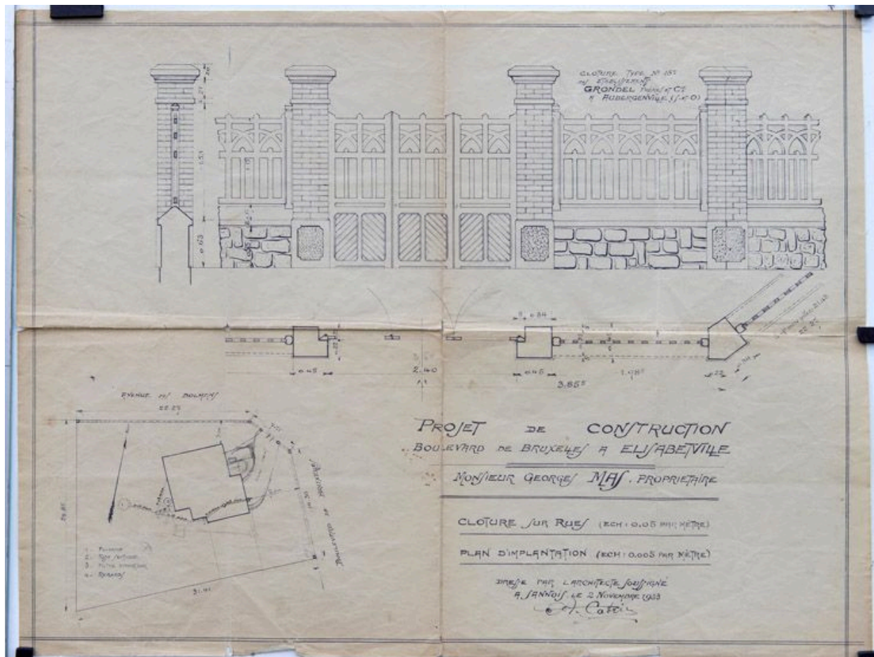
Plan de localisation et dessin des barrières. Tirage. (Collection particulière).
