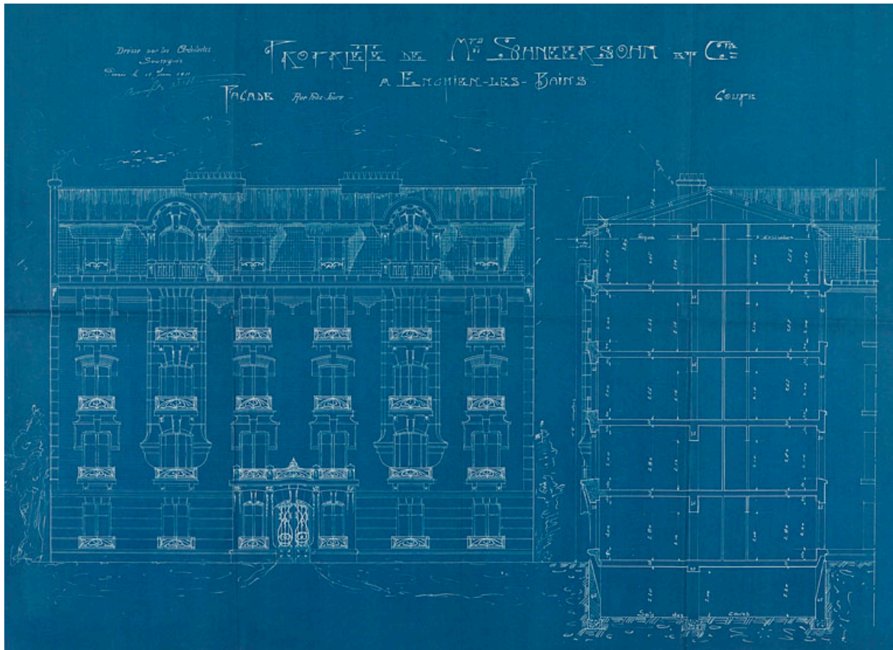
Élévation et coupe d'un immeuble construit en 1911 pour la Société Schneersohn (non localisé). (AM Enghien-les-Bains, Fonds des autorisations de permis de construire)
