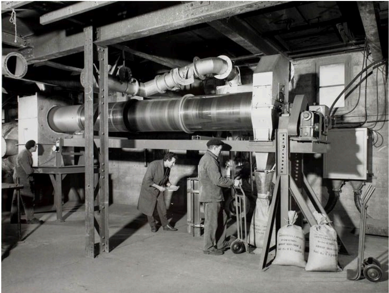
Vue intérieure de la station d'essai, essai de séchage de sable pour four rotatif. Photographie. (AD Seine-et-Marne, 256J3)
