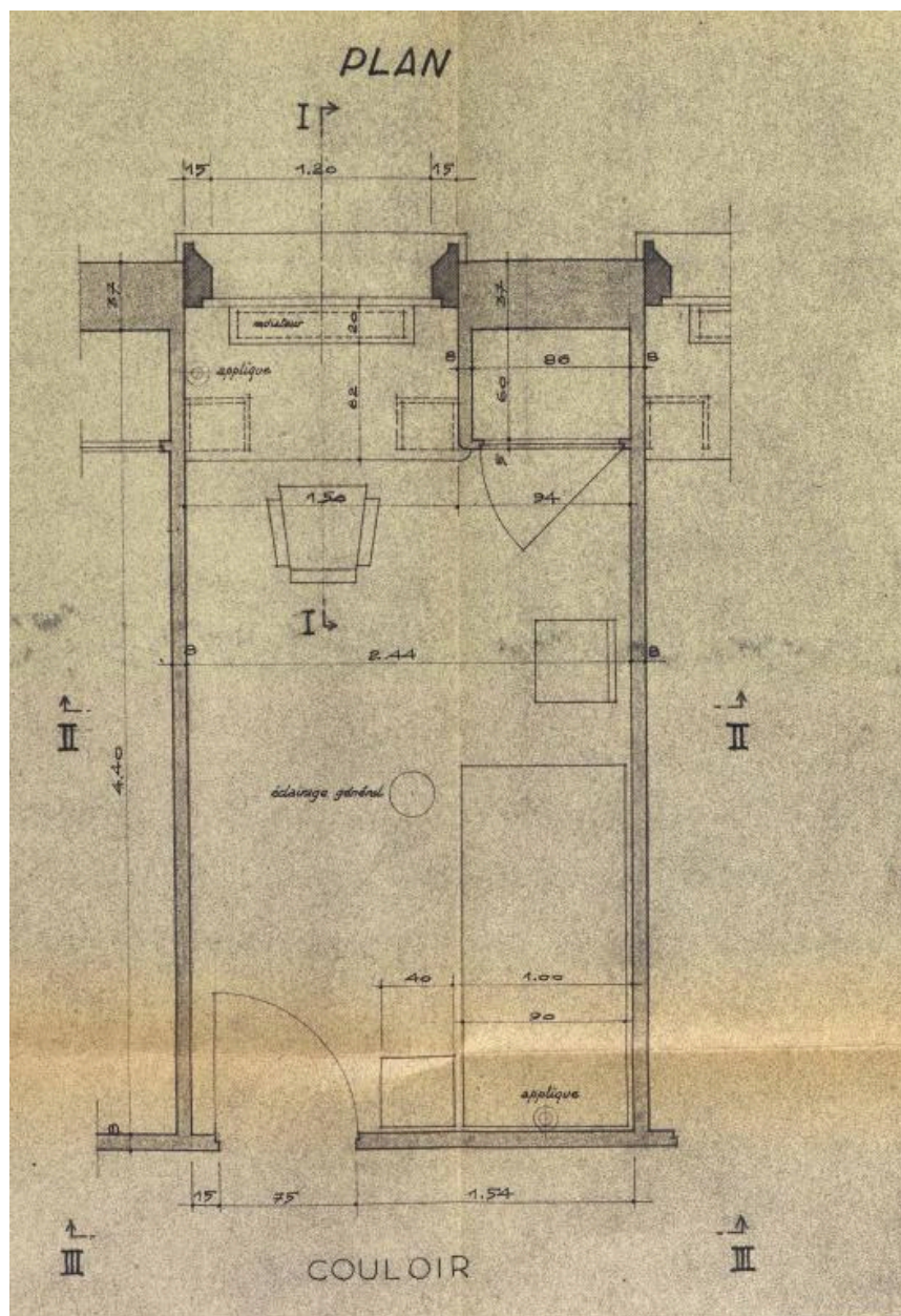
Plan d'une chambre type du pavillon Zellidja ; Jean Walter, architecte ;17 février 1950. Plan. Archives nationales, 20090013/393.
