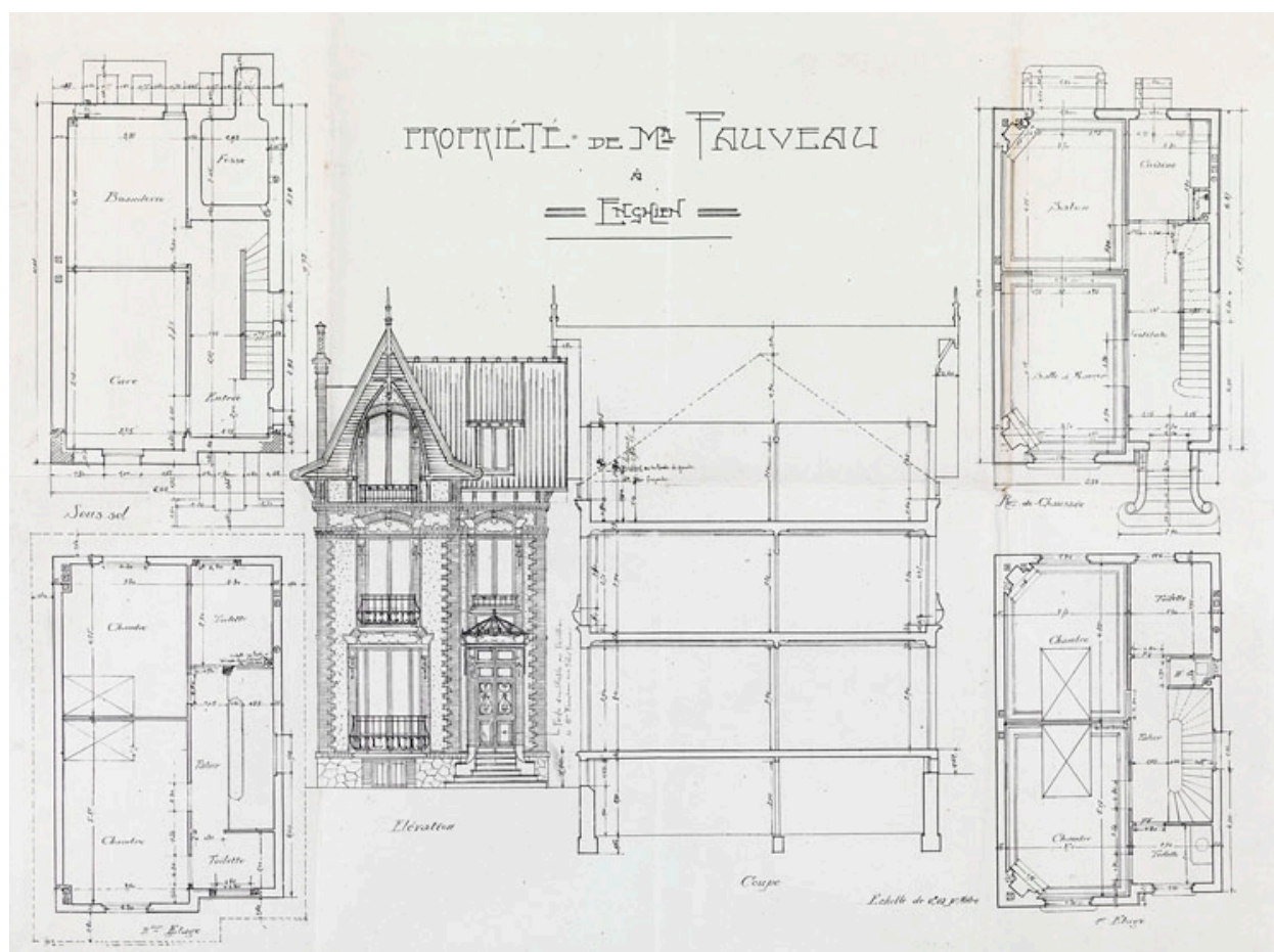
Plans et élévation de la maison construite pour M. Fauveau vers le début du siècle. (AM Enghien-les-Bains, 1T 97)
