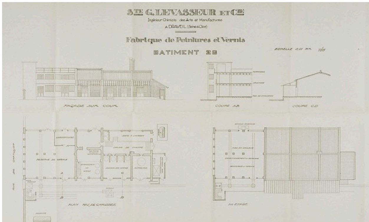
Plan du bâtiment 26 (réserve et cuisson de vernis) : façade, coupe, rez-de-chaussée et 1er étage. 1935. (AD Essonne, 5 M 72)
