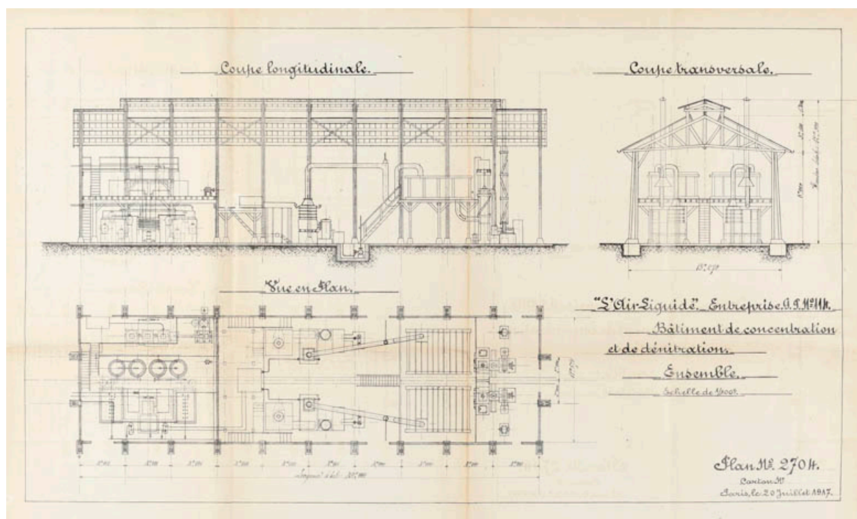
Plan N°2704. 20 juillet 1917. Bâtiment de concentration et de dénitrification. Coupe longitudinale, coupe transversale et vue en plan.
