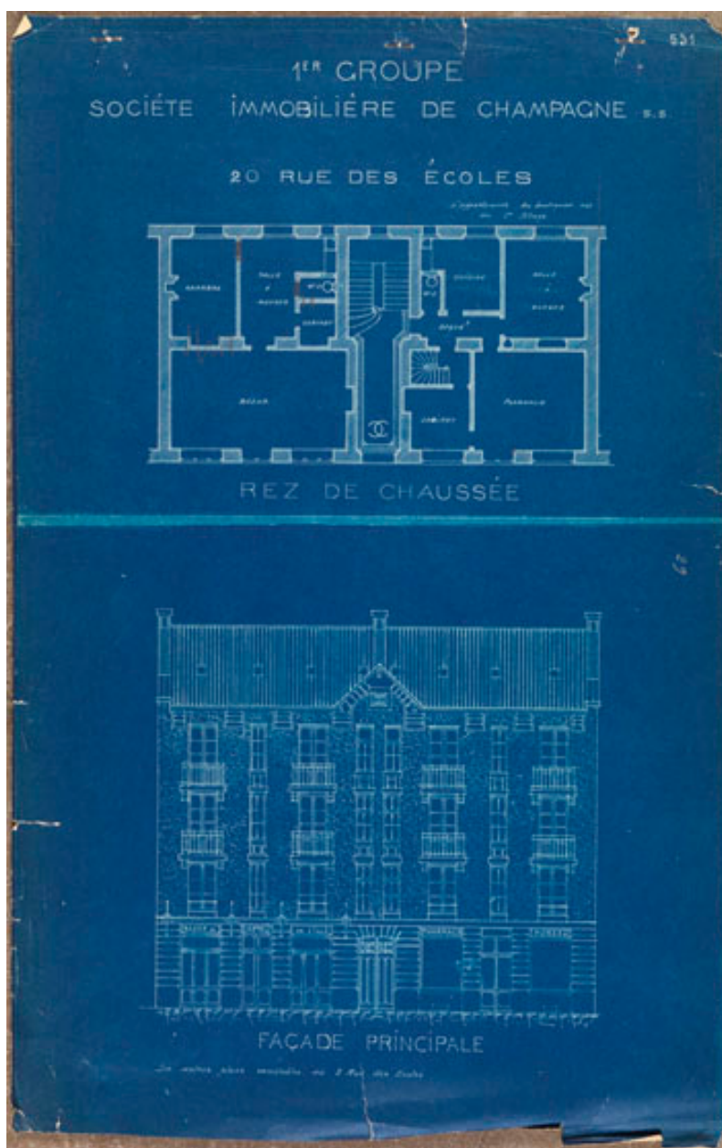
Plan. Société immobilière de Champagne. Façade principale et rez-de-chaussée. 20 rue des écoles.
