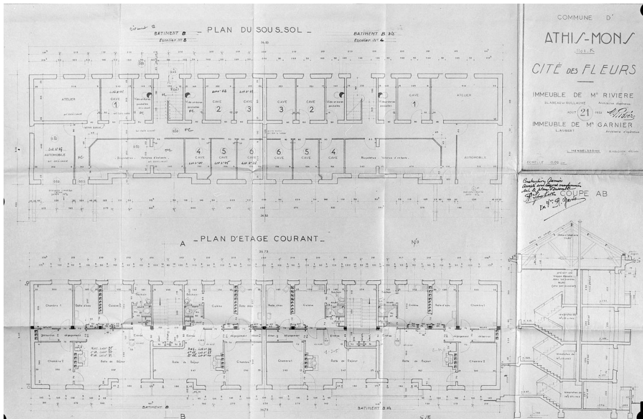
Plan de l'immeuble Rivière et Garnier, dressé par les architectes Blareau, Guillaume et Aubert, août 1953 : sous-sol, étage courant et coupe AB.
