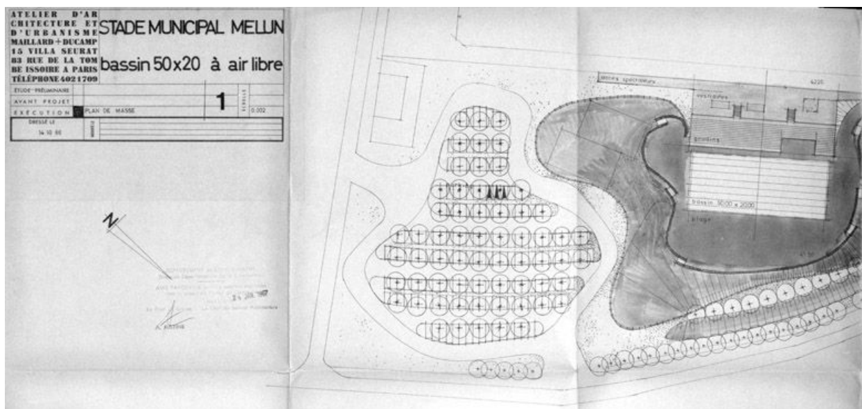
Bassin découvert : plan de situation (partie gauche du document). Tirage d'architecte, 14 octobre 1966. (AM Melun. 466 W 84)
