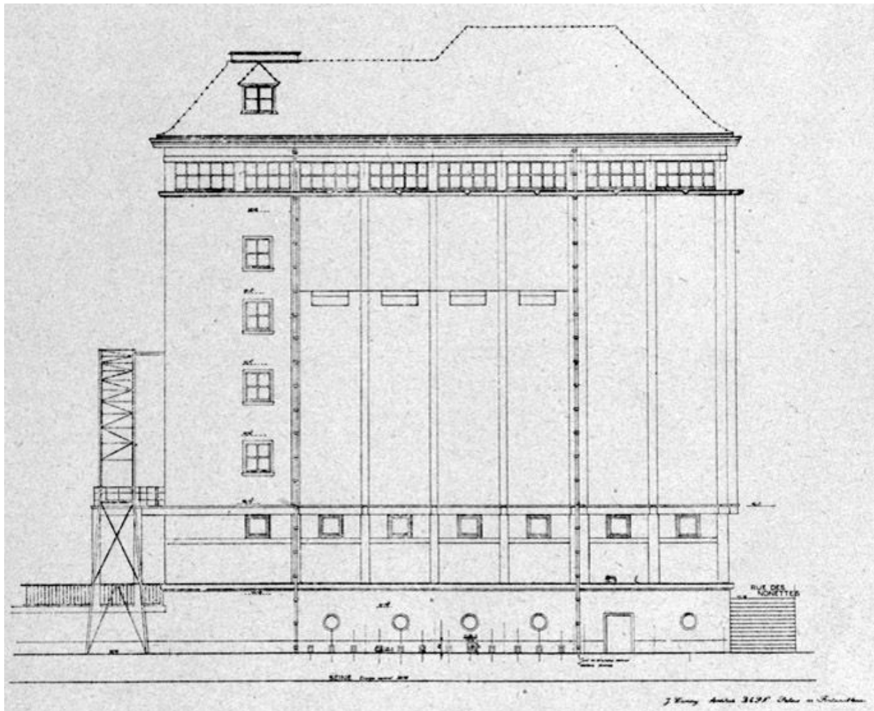
Façade des silos sur la Seine. Photogravure, 1949. Tiré de : L'Architecture française, constructions industrielles (II), n° 85-86, 1949. (AM Melun. 578 W 3)
