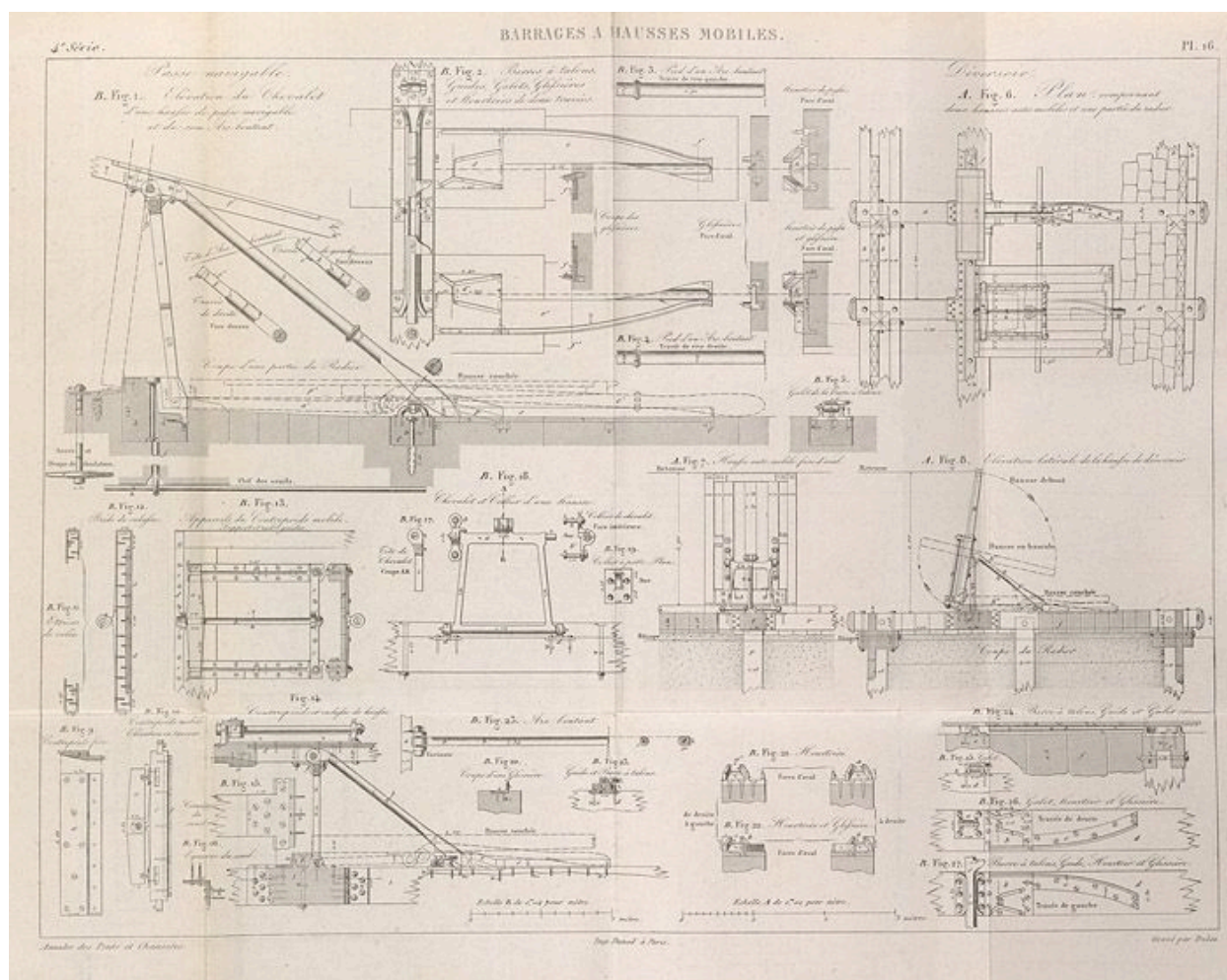
Barrages à hausses mobiles. Elevations et coupes. Tiré de : Mémoire sur les barrages à hausses mobiles / M. Chanoine et M. de Lagrené. In Annales des Ponts et Chaussées, 2e semestre, 1861, n° 21, pl. 15-17.
