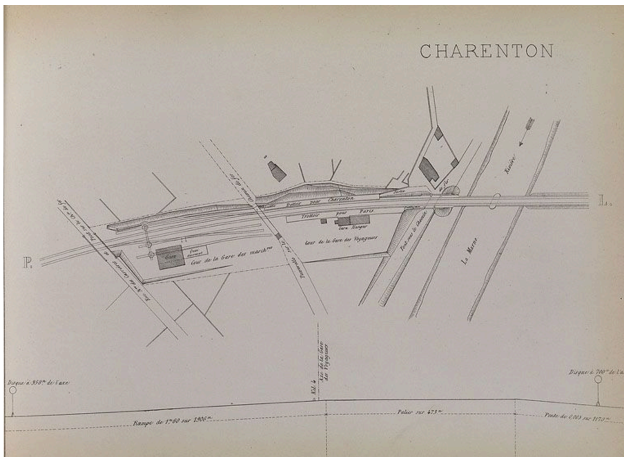
Chemin de fer de Paris à Lyon. Profil général de la ligne ; plans et profils détaillés des gares, s.d. [vers 1852-55], [d'après Lagrière, ancien chef de gare de Bercy]. Plan de la gare de Charenton. (Ecole nationale des ponts et chaussées)
