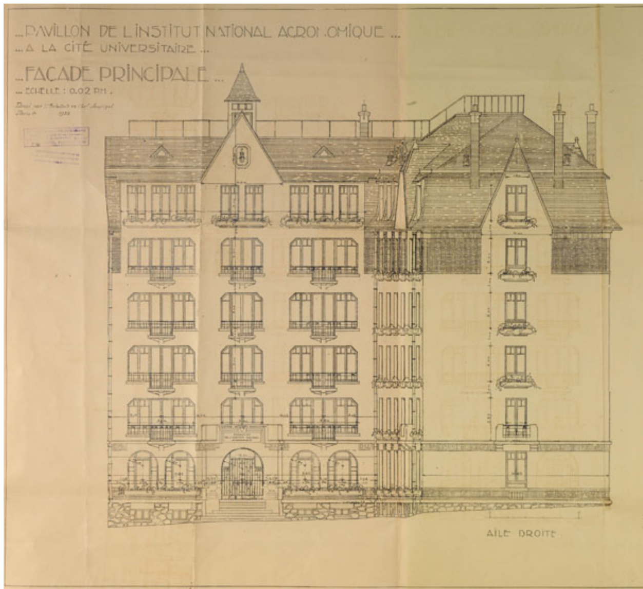
Élévation principale (partie centrale et aile droite), par l'architecte René Patouillard-Demoriane. 1928. Plan. Archives nationales, 20090013/385.
