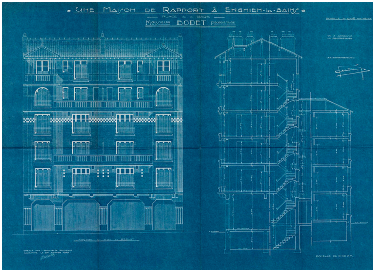
Élévation et coupe de l'immeuble construit pour monsieur Bodet en 1929, place de la Gare. (AM Enghien-les-Bains, Fonds des autorisations de permis de construire)
