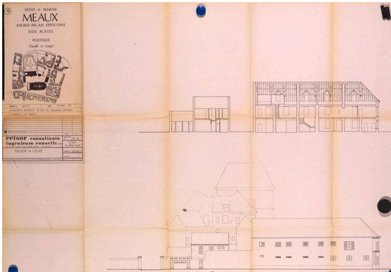
La posterie (bâtiment de communs, le long de la rue Bossuet) : façade et coupe. (Musée Bossuet, Meaux)
