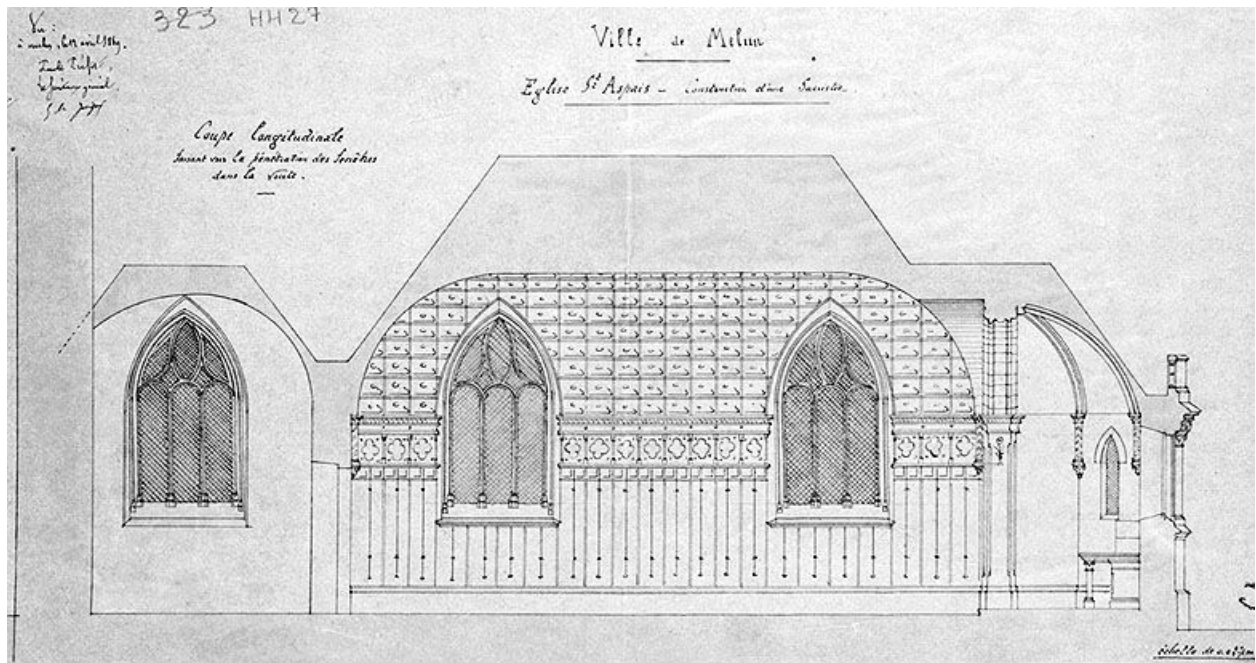
Ville de Melun. Eglise Saint-Aspais. Construction d'une sacristie. Coupe longitudinale. Echelle : 0.02 m.p.m. Calque aquarellé, 1869. (BM Melun. HH 27)
