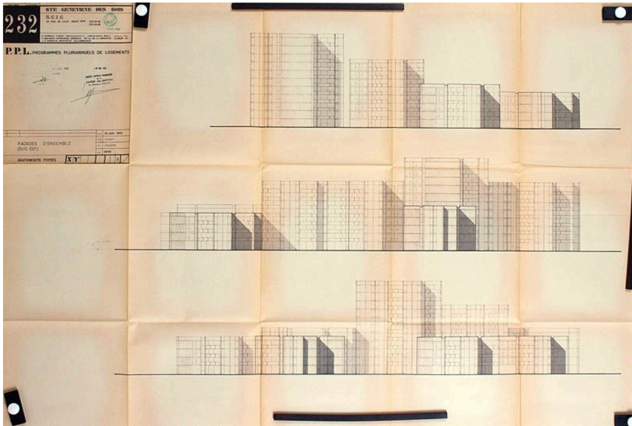
cité dite Résidence Pergaud. Elévation des façades d'ensemble.
