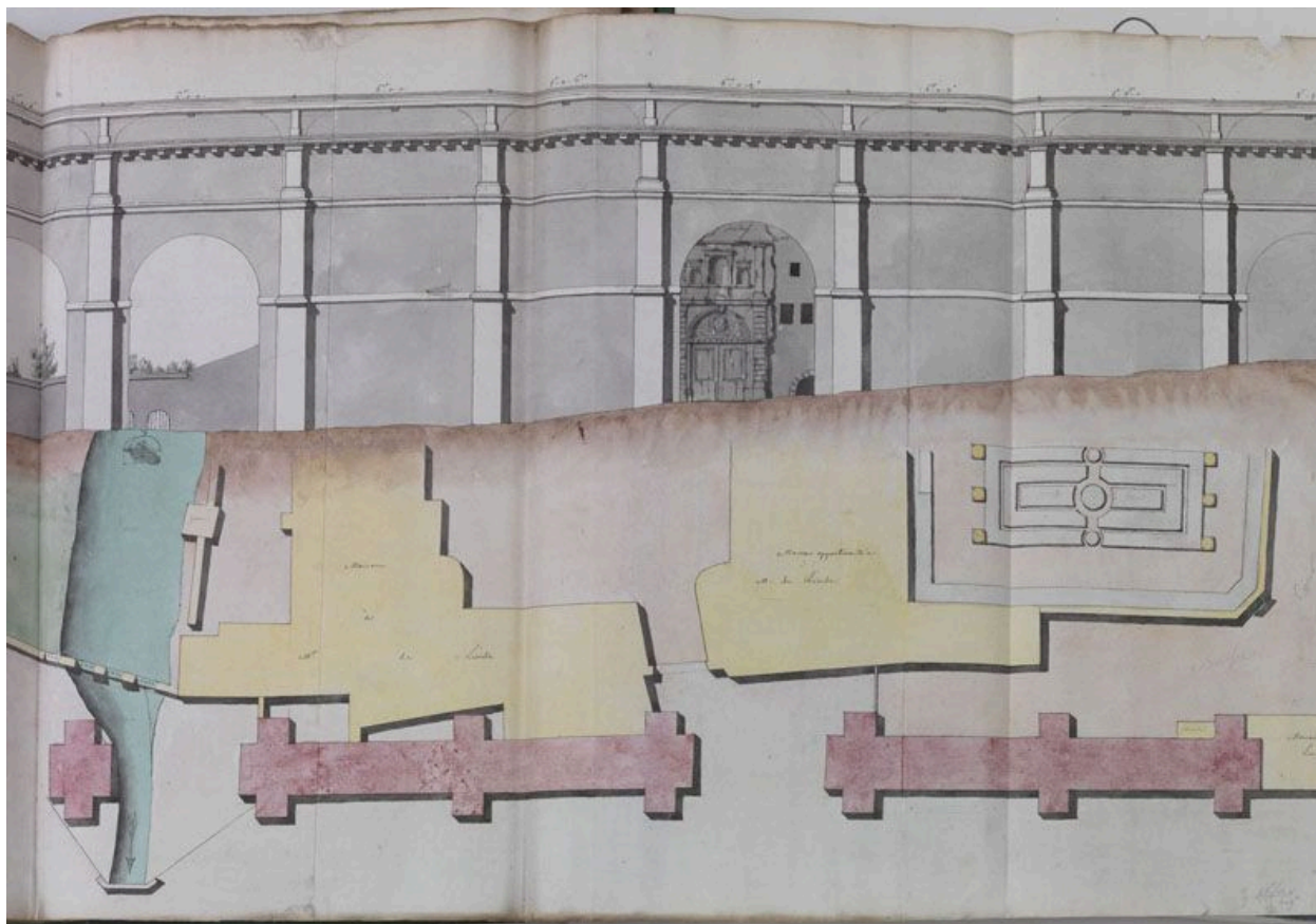
Arcueil. Elévation et plan du pont-aqueduc d'Arcueil avec les noms des propriétés jouxtant l'édifice (18e siècle) : sous le pont, façade de la Maison Renaissance du Fief des Arcs et d'Anjou. (Bibliothèque de l'Ecole de Nationale des Ponts et Chaussées, Ms.2783)
