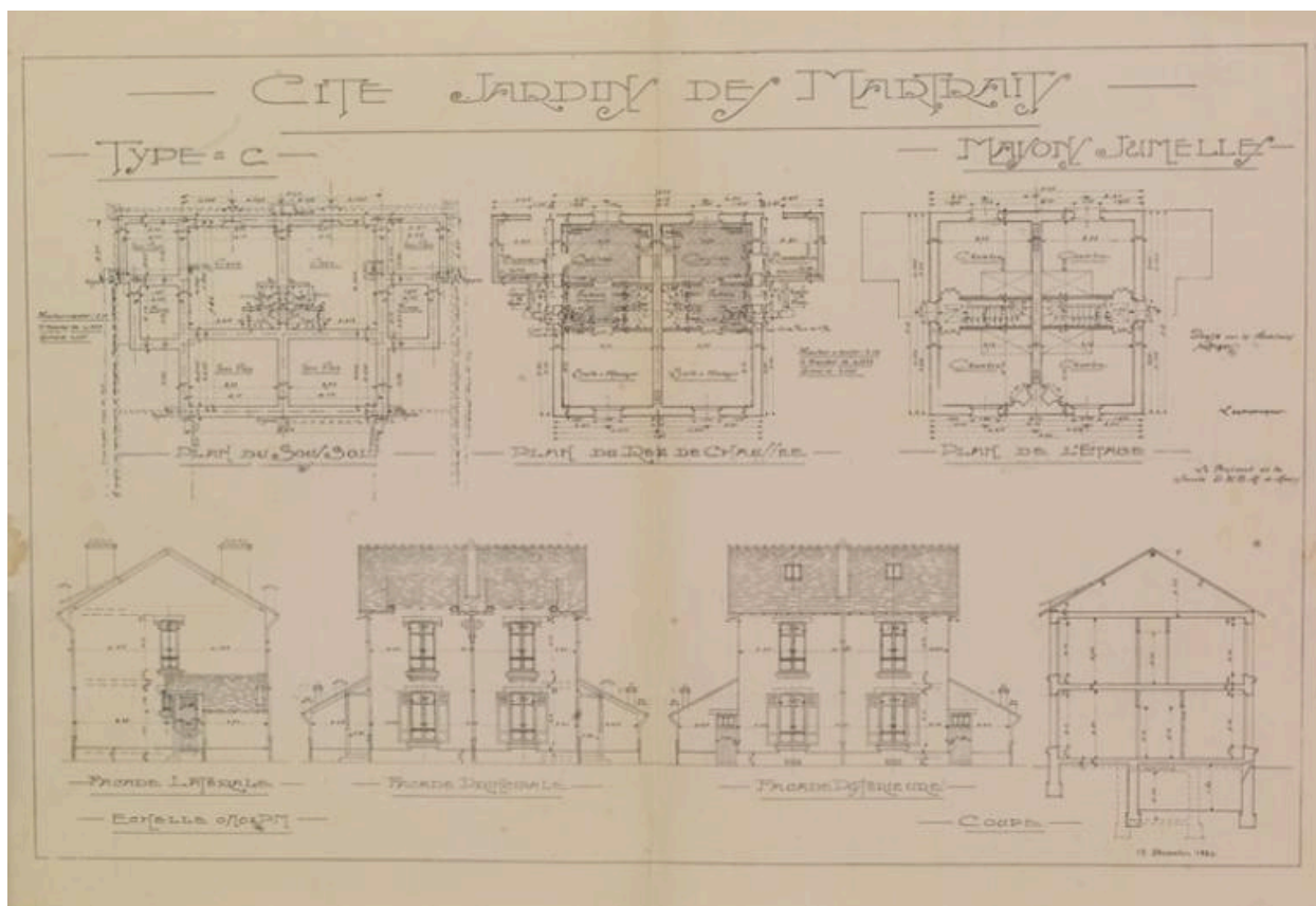
Élévation et plans des maisons jumelles 4-30 avenue Victor Hugo (type C), non signé, 1924 (AM Mantes-la-Jolie, non coté).
