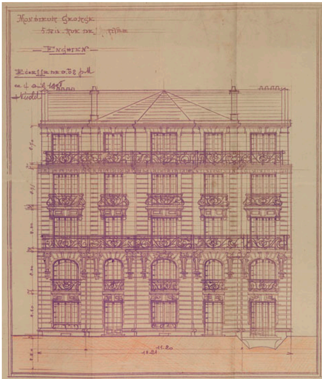
Premier projet d'élévation sur rue de l'immeuble alors dépourvu d'étage de comble (avril 1908) (AM Enghien-les-Bains, 1T 8)
