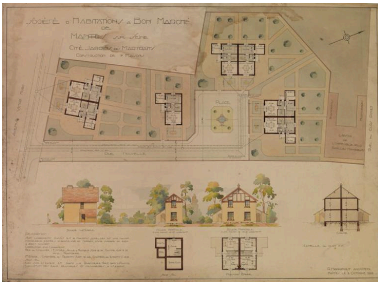
Plan et élévations des maisons impasse Victor Hugo (type B), (non réalisé), Marabout (architecte), 1928 (AM Mantes-la-Jolie non coté).
