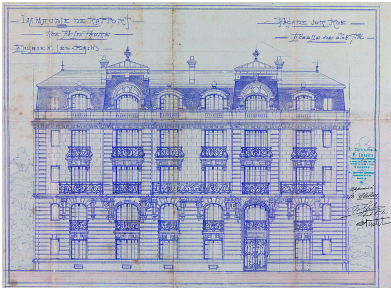
Élévation d'un immeuble conçu pour madame Claudot en 1909. Edifice non localisé. (AM Enghien-les-Bains, Fonds des autorisations de permis de construire)
