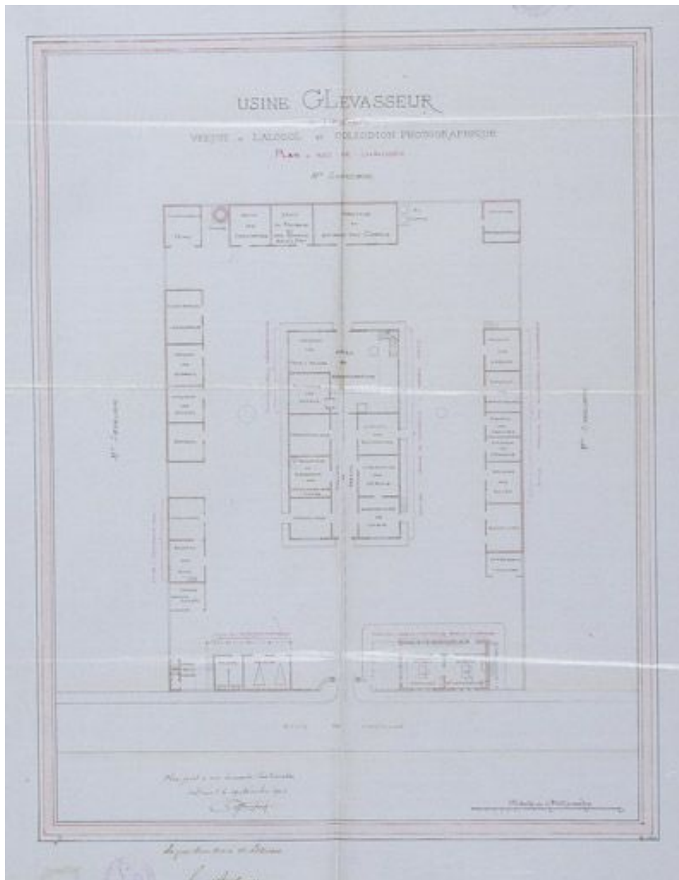
Usine de M. Levasseur (verniss à l'alcool et collodion photographique) : plan du rez-de-chaussée. 19 novembre 1903. (AD Essonne, 5 M 72)
