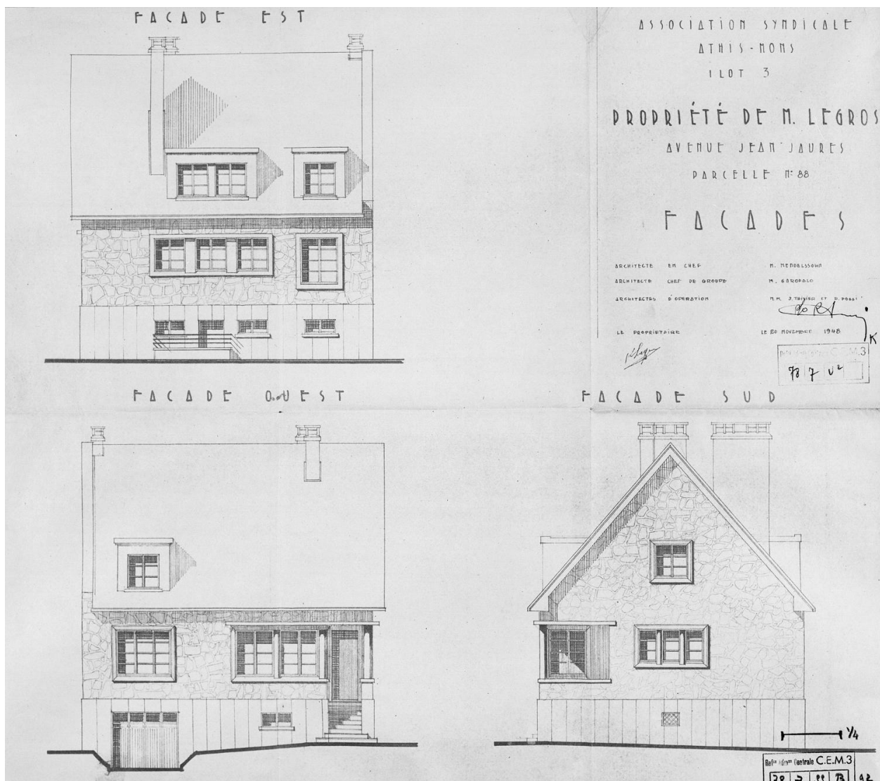
Elévations de la maison reconstruite dans l'îlot 3 (parcelle 88) pour M.Legros (34, avenue Jean-Jaurès) ; architecte en chef Léo Mendelssohn, P. Garofalo, architecte chef de groupe et Thivier et Poggi, architecte d'opération, 20 novembre 1948.
